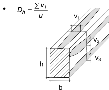
Bild 12: Messung des Druckholzanteils
